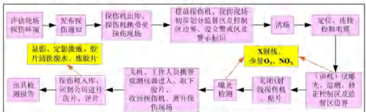
图9-4 移动式X射线探伤工作流程及产污环节
