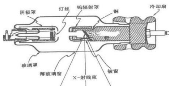
图 9-4 X 射线管结构示意图
