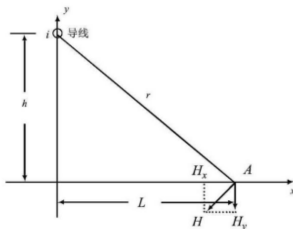
图 3.1-4 磁场向量图
