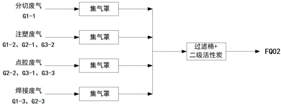
图 5.1-1 废气处理线路图
