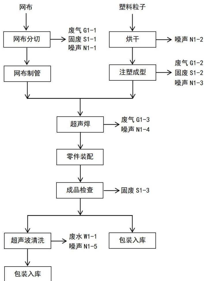
图 2-3 过滤器生产工艺流程及产排污环节 1
