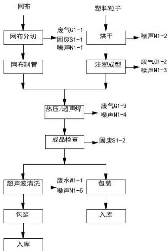
图 2-6 过滤器生产工艺流程及产排污环节 1
