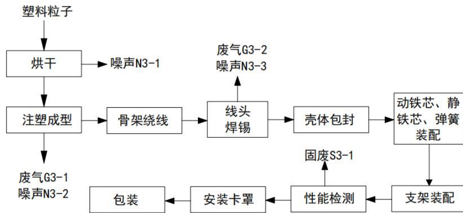
图 2-11 电磁阀生产工艺流程及产排污环节
