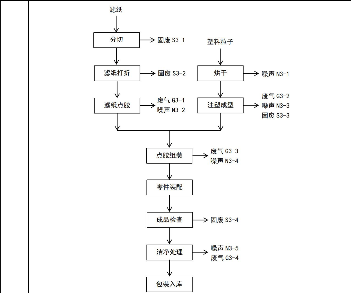
图 2-5 过滤器生产工艺流程及产排污环节 3
