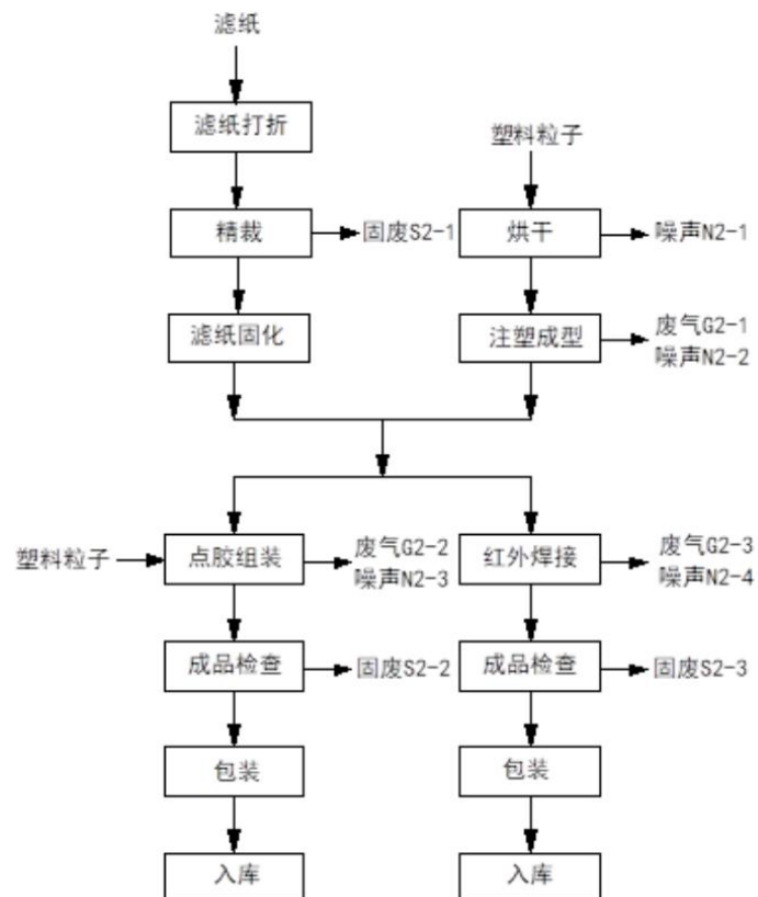
图 2-7 过滤器生产工艺流程及产排污环节 2
