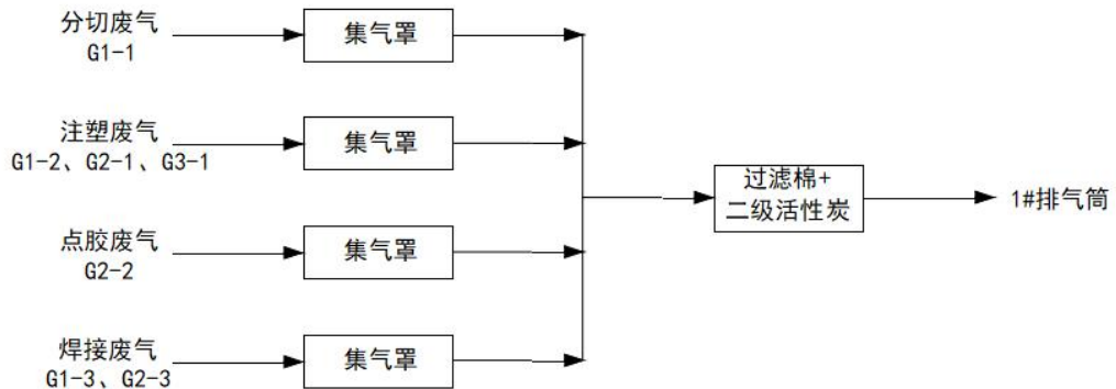
图 2-12 现有项目废气处理工艺流程图
