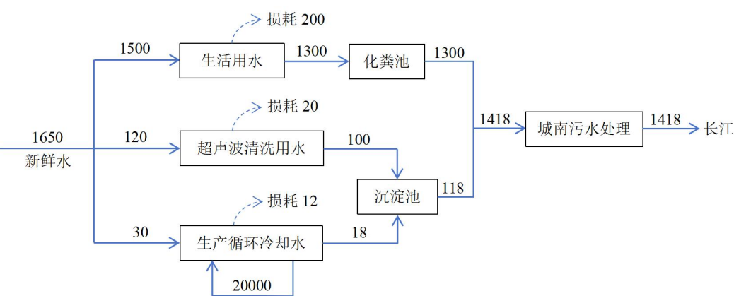
图 2-2 项目建成后全厂水平衡图（单位：t/a）
