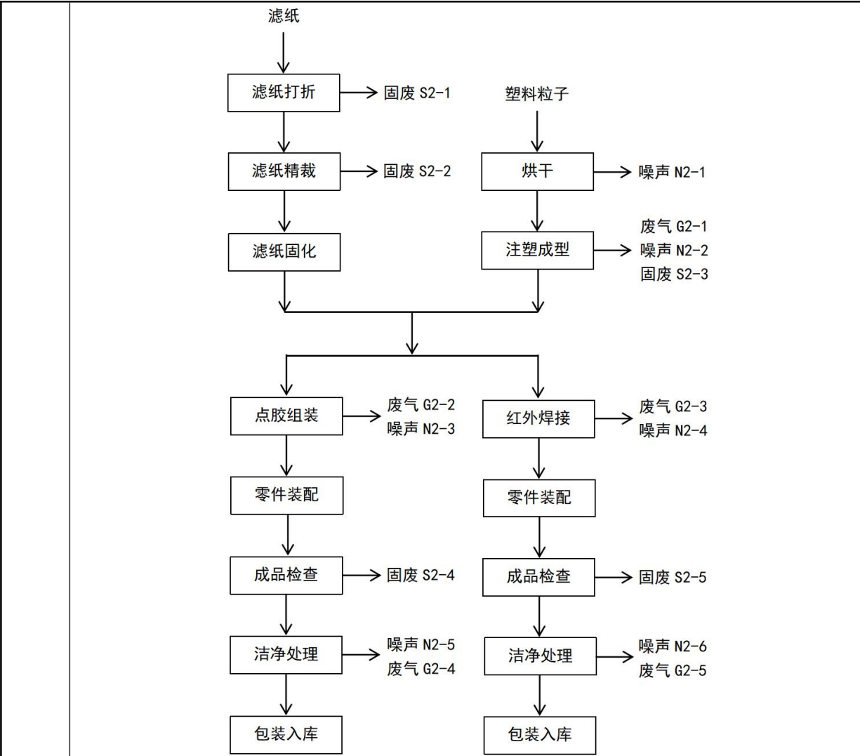
图 2-4 过滤器生产工艺流程及产排污环节 2
