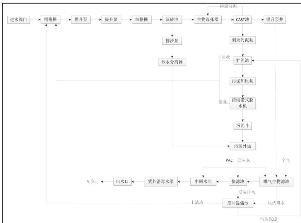
图 4-3 仙林污水处理厂工艺图
