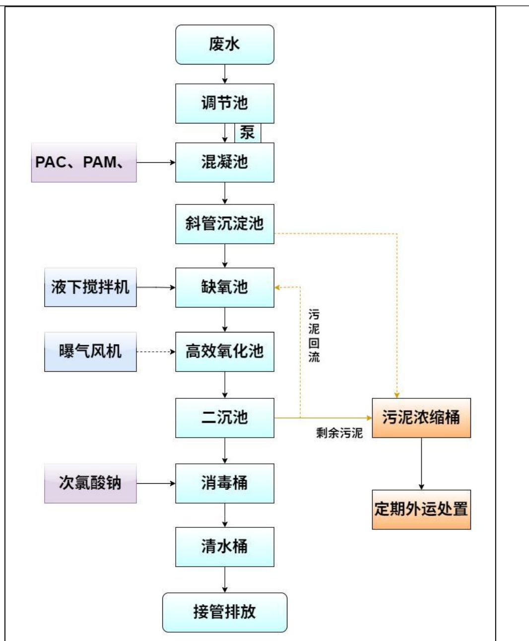
图 4-2 废水处理设施工艺流程图
