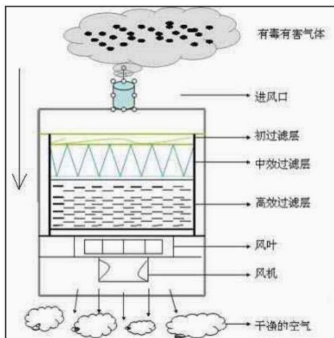
图 4-3 HEPA 工作原理示意图
