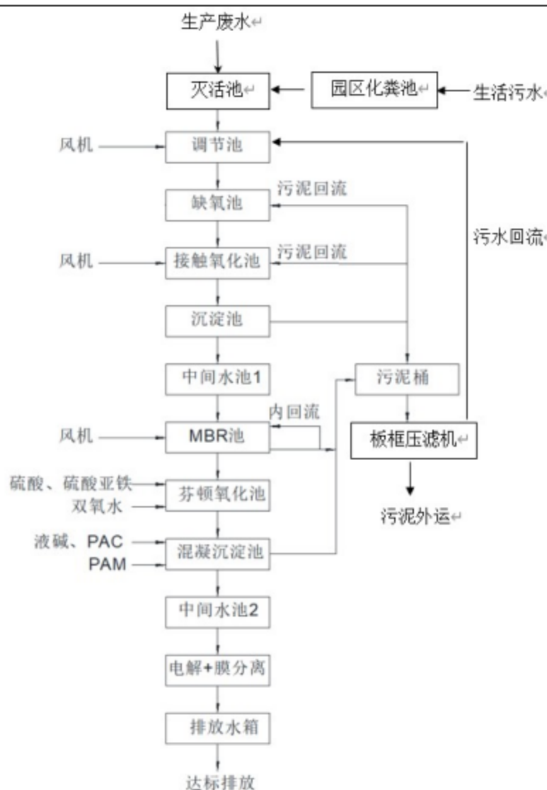
图 4-2 污水处理站工艺流程图
