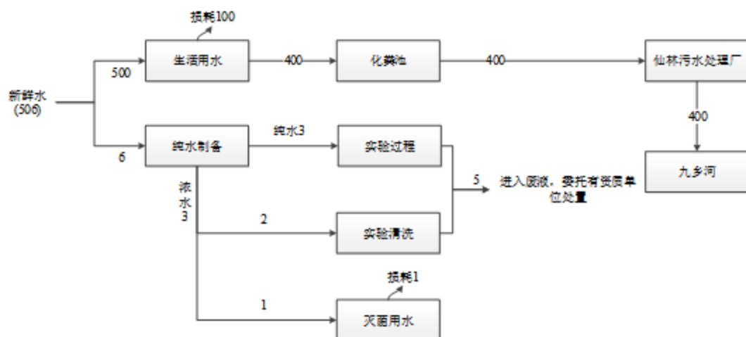
图 2-5 现有项目水平衡图
