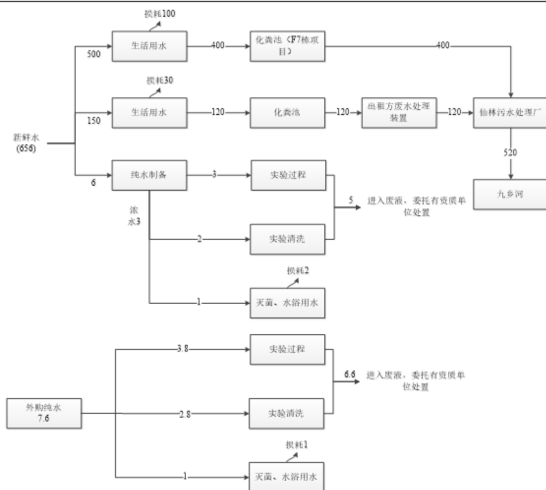
图 2-2 扩建后全厂水平衡图 (t/a)
