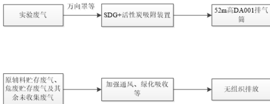
图 5.1.1-1 废气收集、处理示意图
