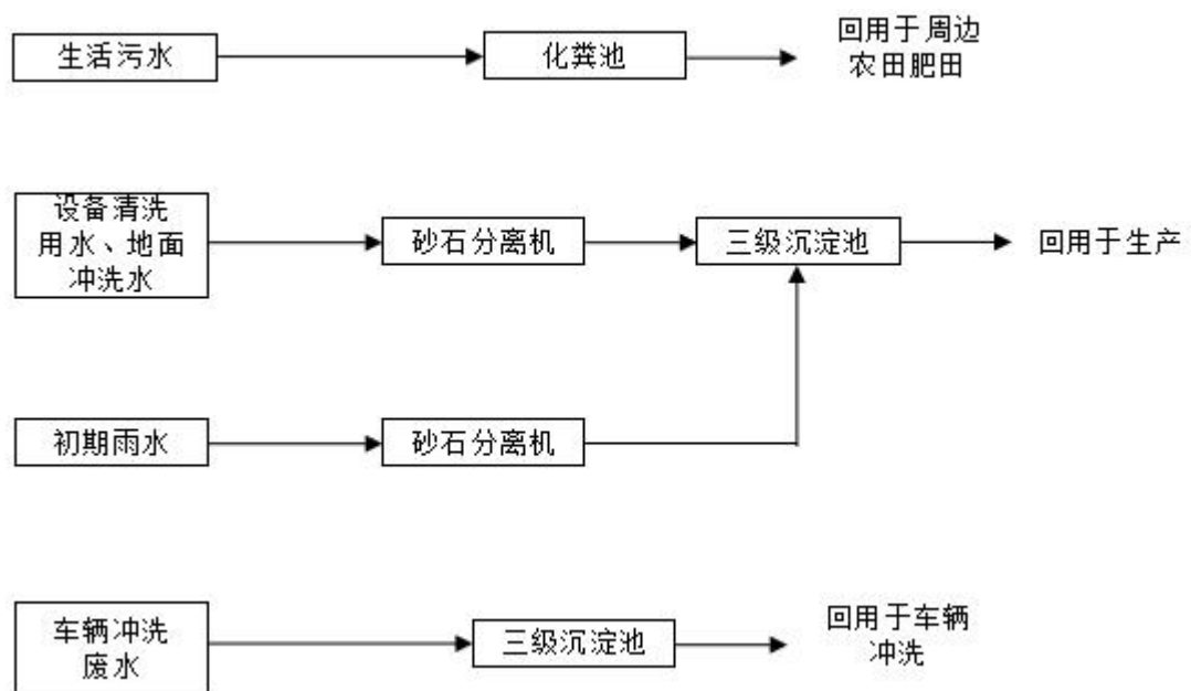
图 4-3 本项目废水收集、处理方式示意图
