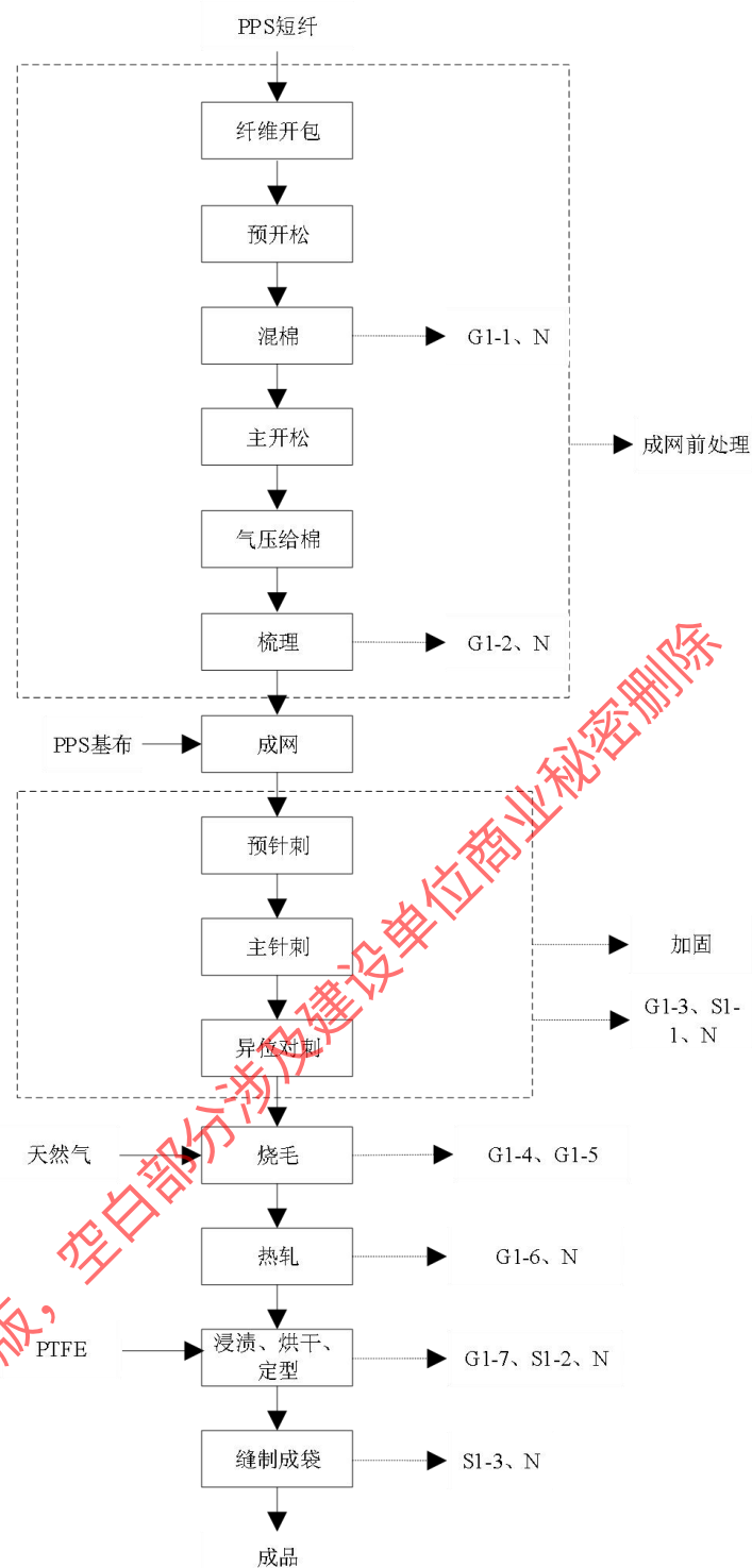
图 2.3-1 滤袋生产工艺流程图
