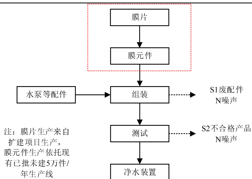
图 2.2-2 净水装置总体生产工艺流程
