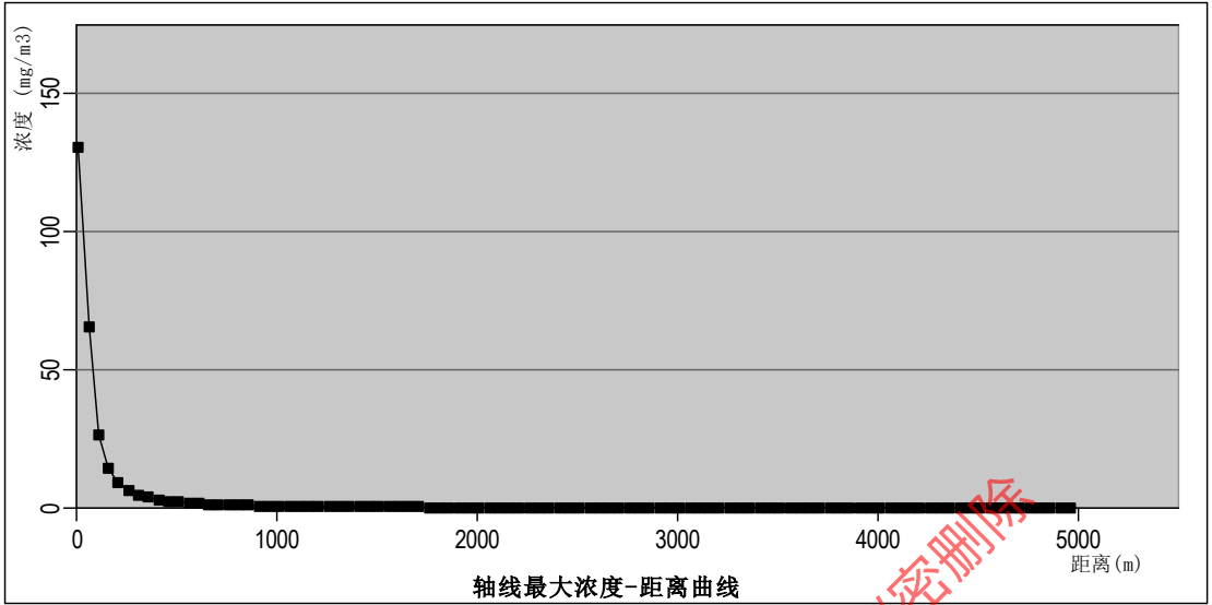
图 6.1-1 最不利气象条件风向不同距离出 N,N-二甲基甲酰胺（DMF）最大浓度预测结果图
