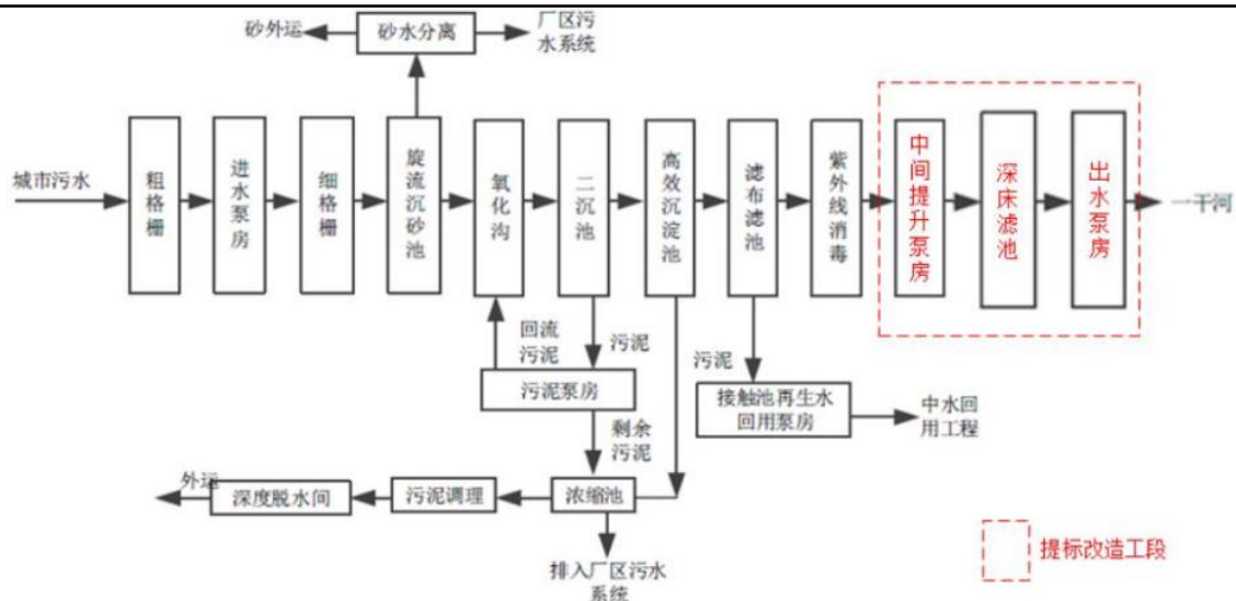
图 4.1-5 南京溧水秦源污水处理有限公司污水处理工艺流程图（一、二期）
