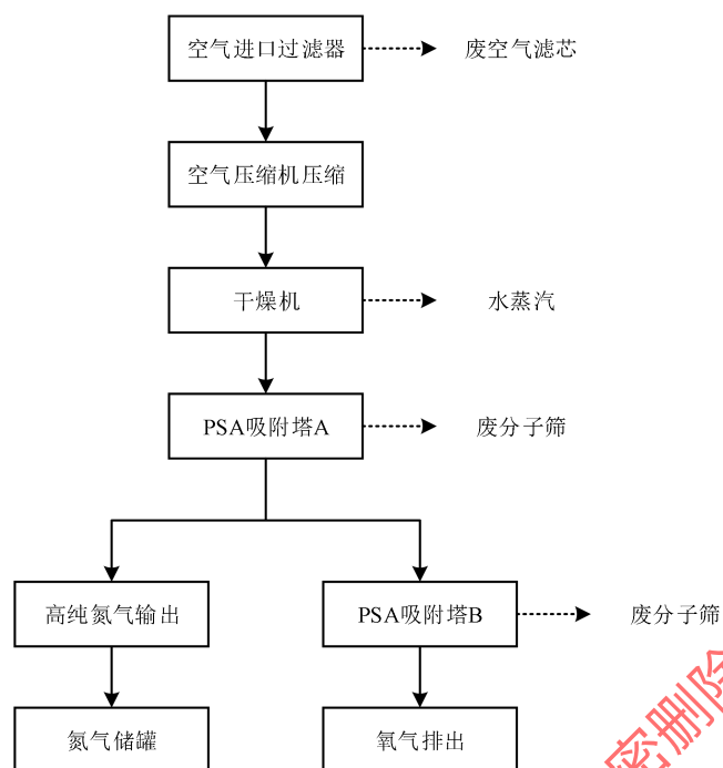
图 2.2-4 分子筛脱附工艺制氮工艺流程图
