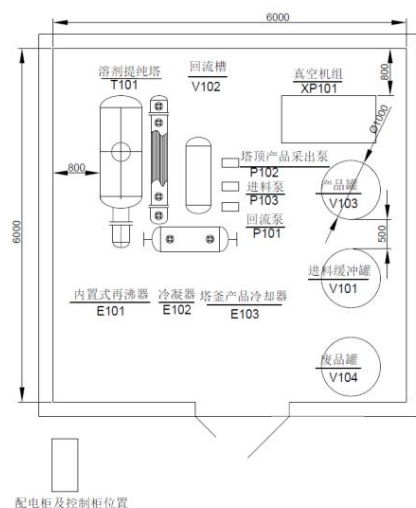
图 2.2-5 油相溶剂回收装置内部系统图
