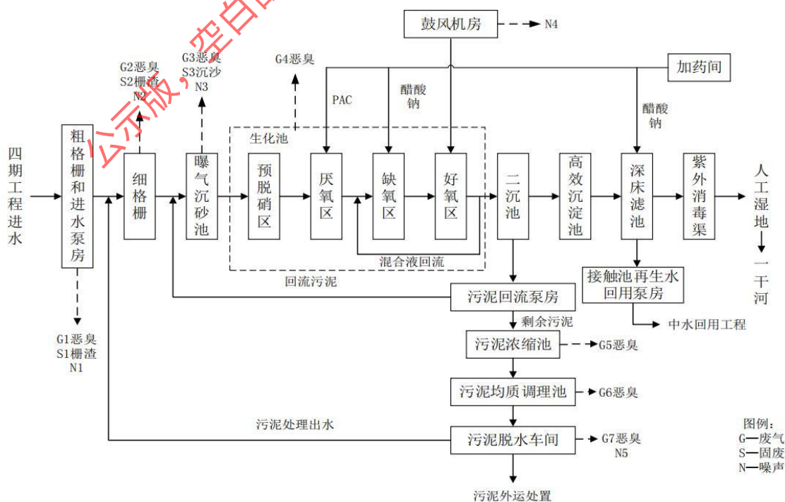
图 4.1-7 南京溧水秦源污水处理有限公司污水处理工艺流程图（四期）
