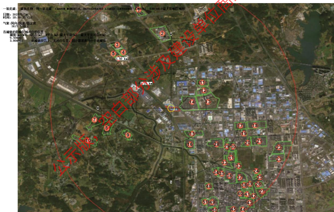
图 6.1-6 最不利气象条件风向不同距离 CO 最大影响区域图
