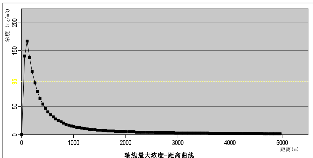
图 6.1-3 最不利气象条件风向不同距离出 CO 最大浓度预测结果图
