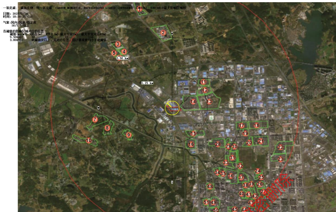
图 6.1-5 最不利气象条件风向不同距离 CO 最大影响区域图
