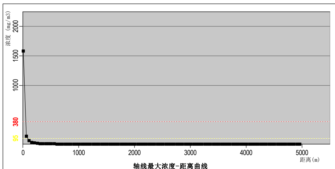
图 6.1-7 最不利气象条件风向不同距离出 CO 最大浓度预测结果图
