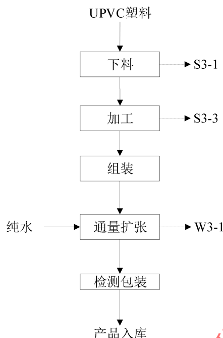
图 2.3-3 PVDF 中空纤维膜组件生产工艺流程图
