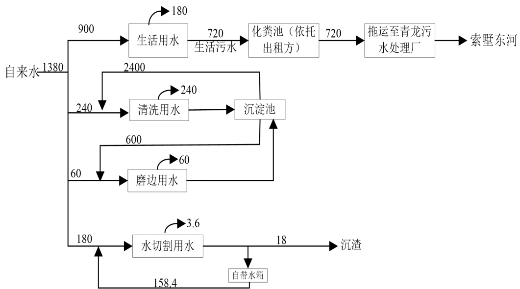
图 2-2 项目全厂水平衡图 (单位: t/a)
