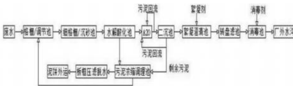
图 4-1 青龙污水处理厂工艺流程图
