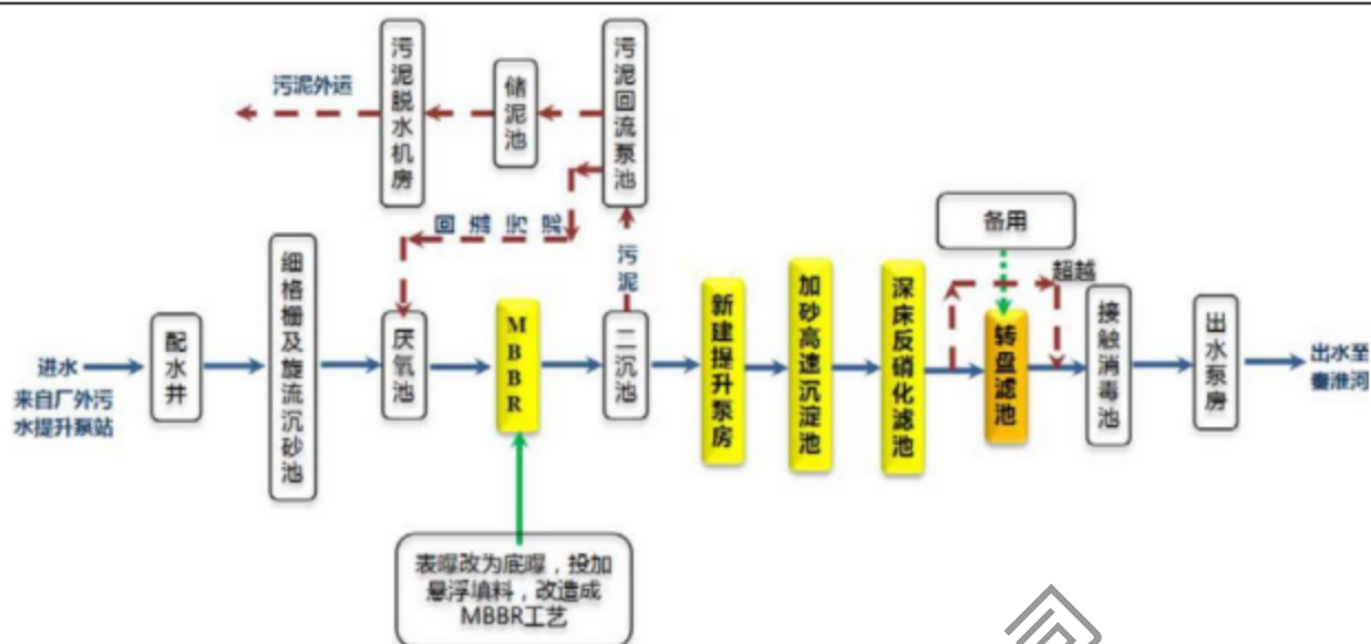
图 4-1 江宁高新区污水处理厂提标改造后污水处理工艺流程图
