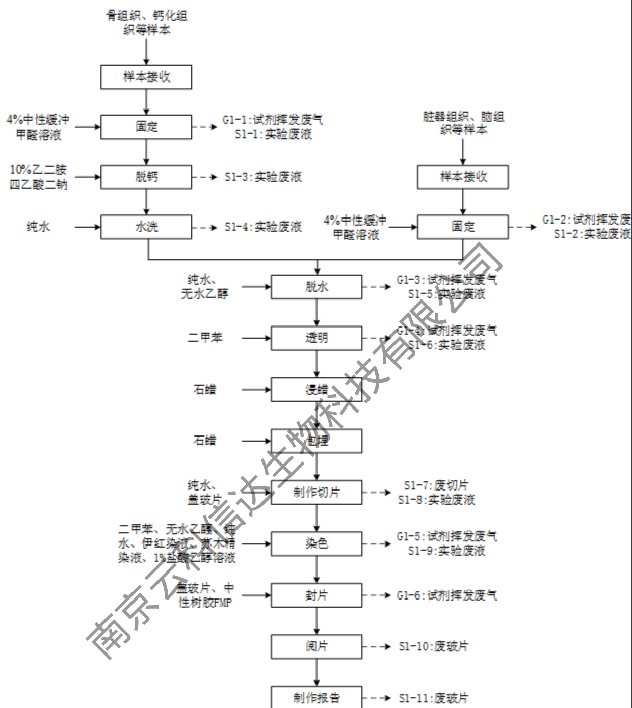
图 2-2 病理检测实验工艺流程图
