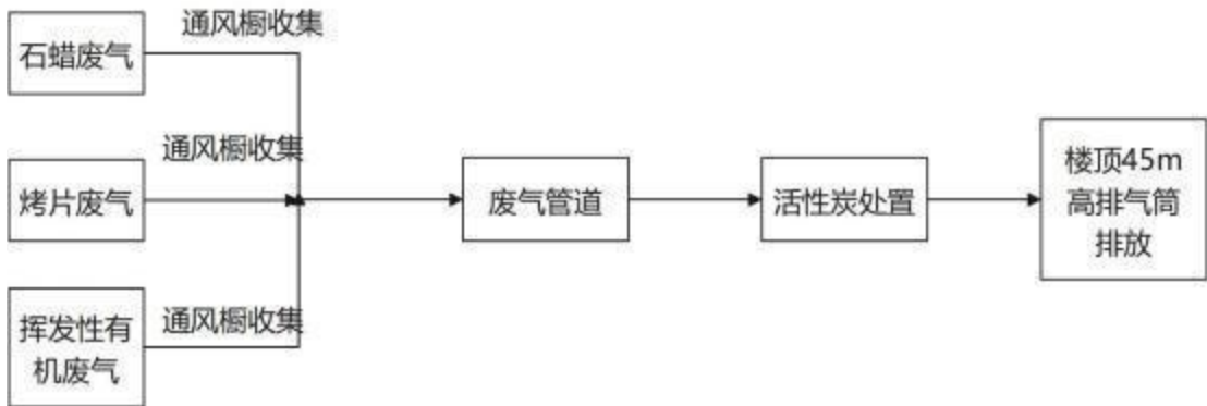
图4-1本项目废气治理示意图
