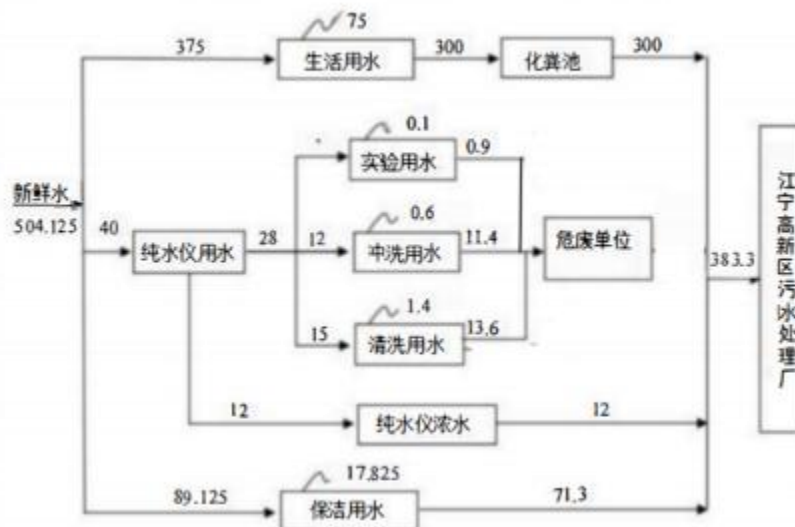
图2-1项目用水平衡图（单位：t/a）
