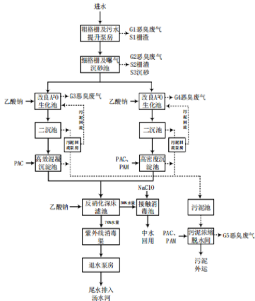
图 4-3 江宁汤山新城污水处理厂提标改造后污水处理工艺流程图
