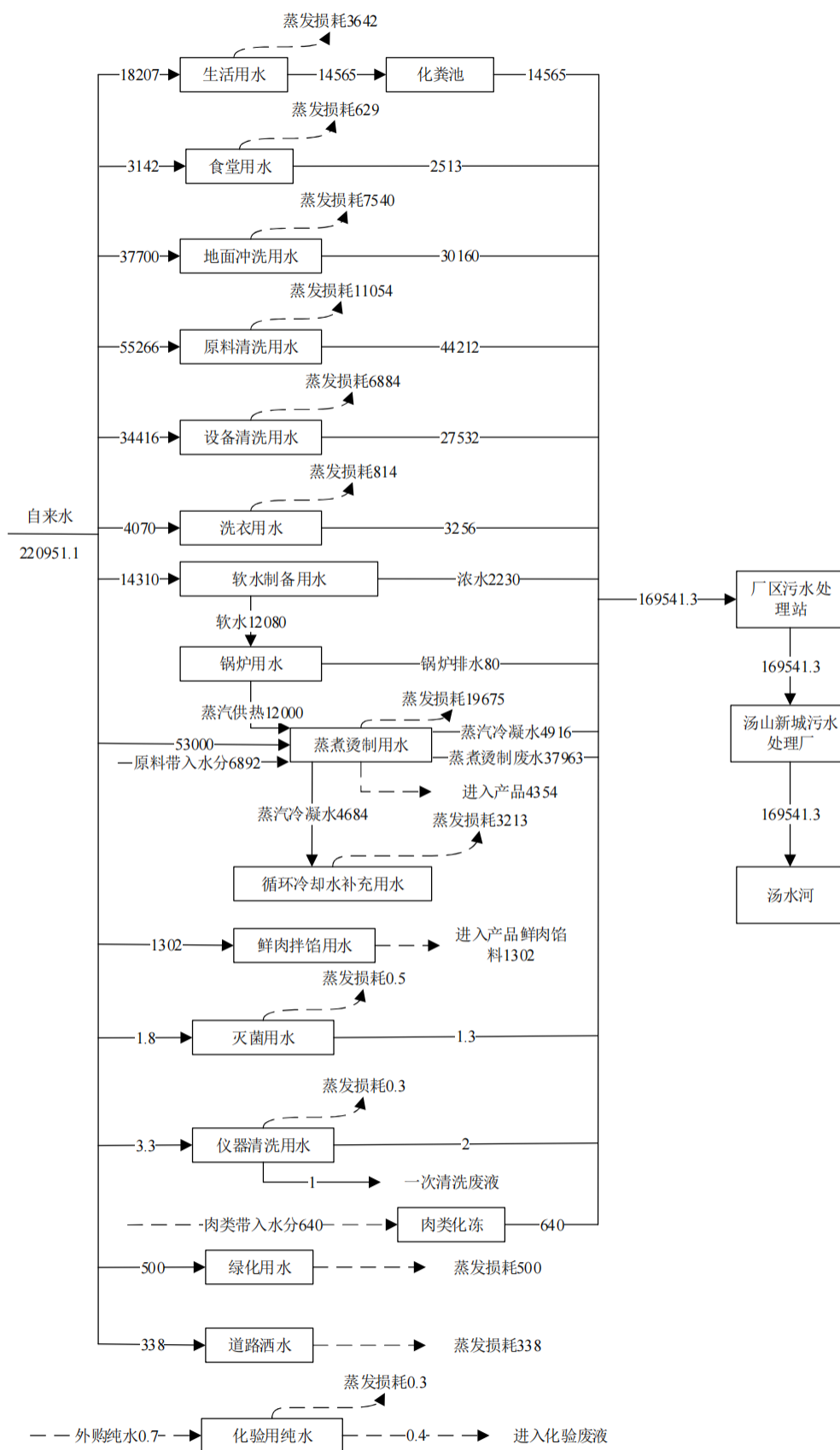
图 2-2 本项目运营后全厂用水平衡图
