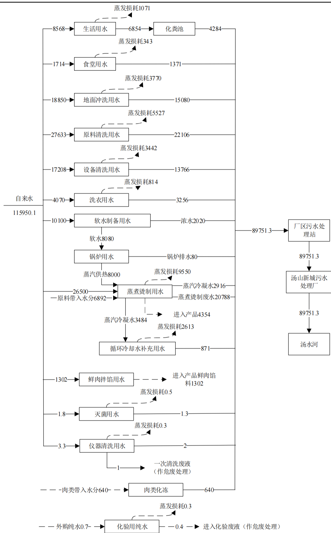
图 2-1 本项目用水平衡图
