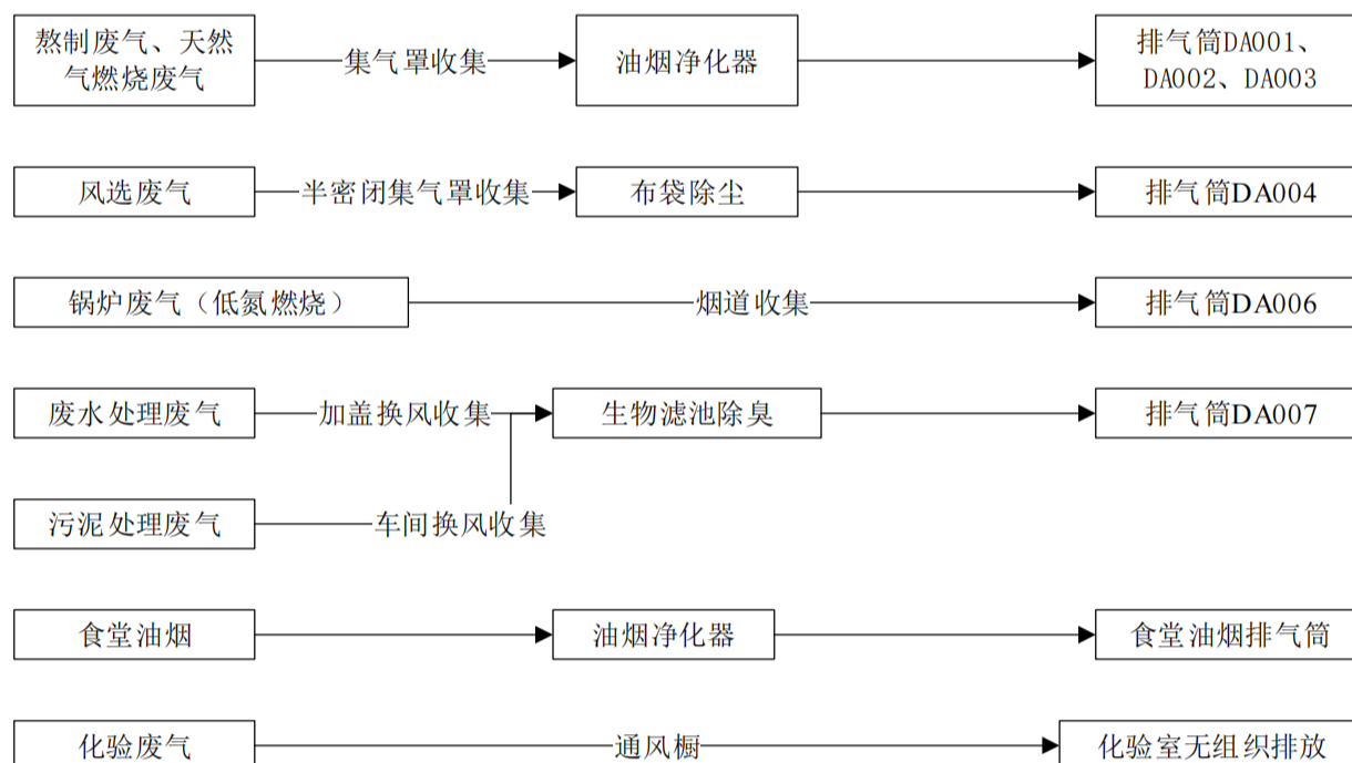
图 4-1 废气收集处理示意图
