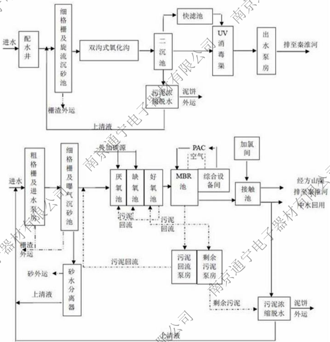
图 4-1 江宁科学园污水处理厂处理工艺流程图
