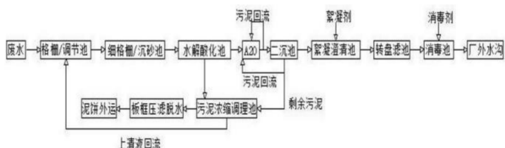
图4-3 青龙污水处理厂工艺流程图
