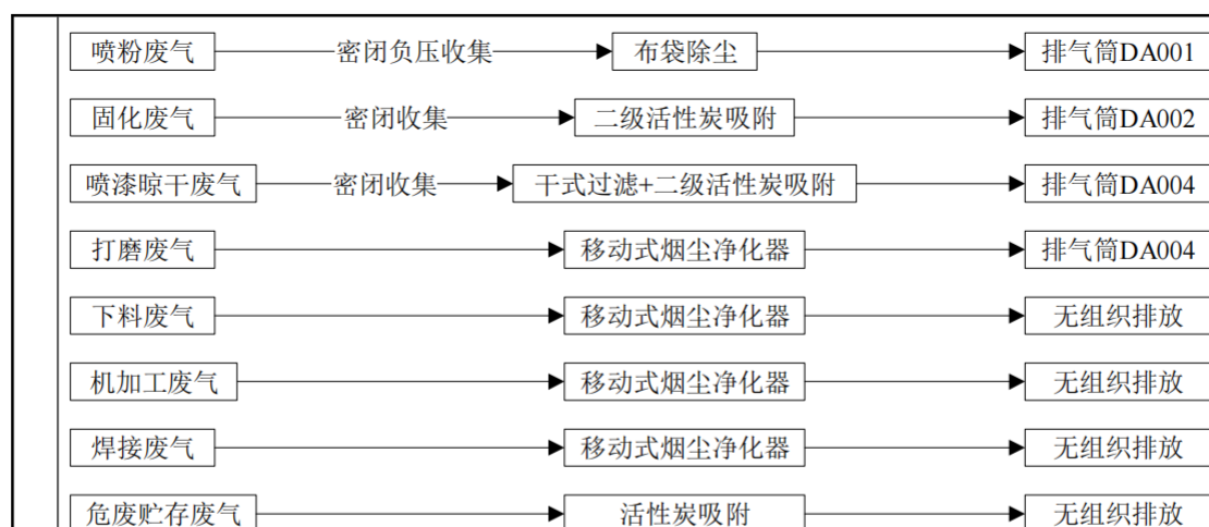
图4-1 废气走向流程图
