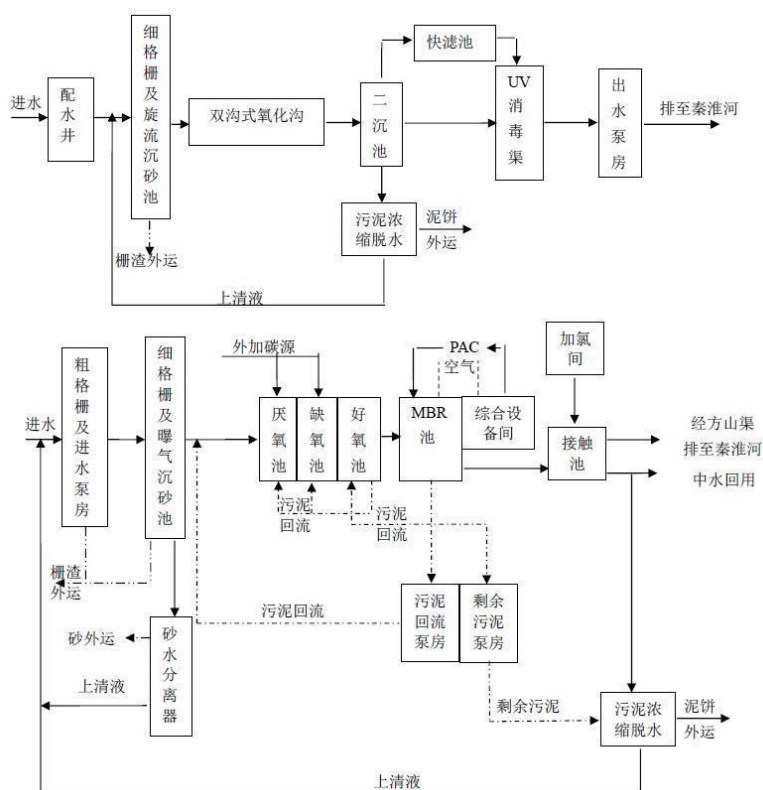
图 4-1 科学园污水处理厂污水处理工艺流程图
