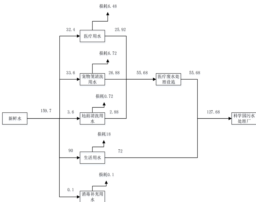
图 2-1 建设项目水平衡图 (单位: t/a)
