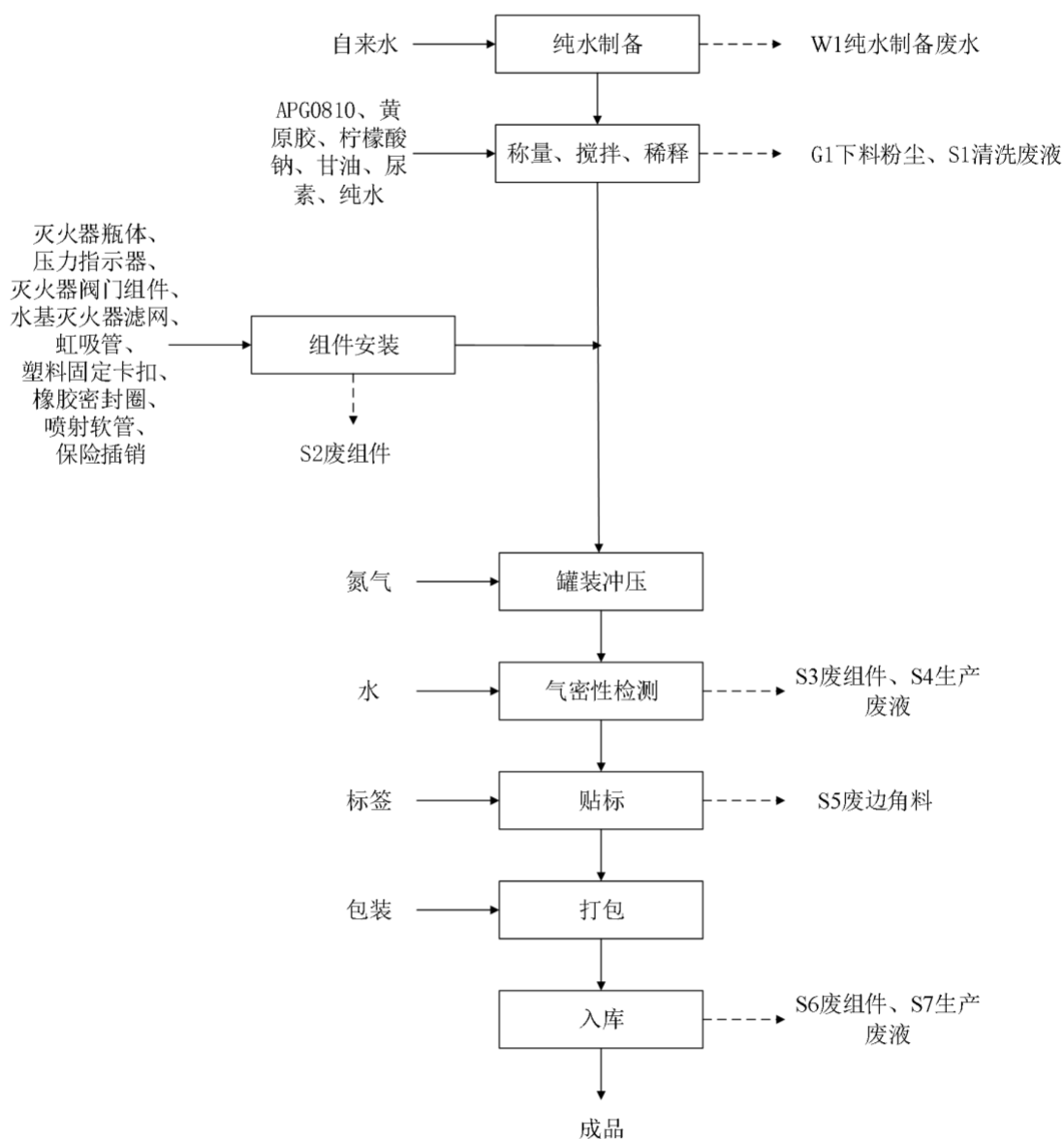
图 2-2 水基型灭火器生产工艺流程及产污环节图
