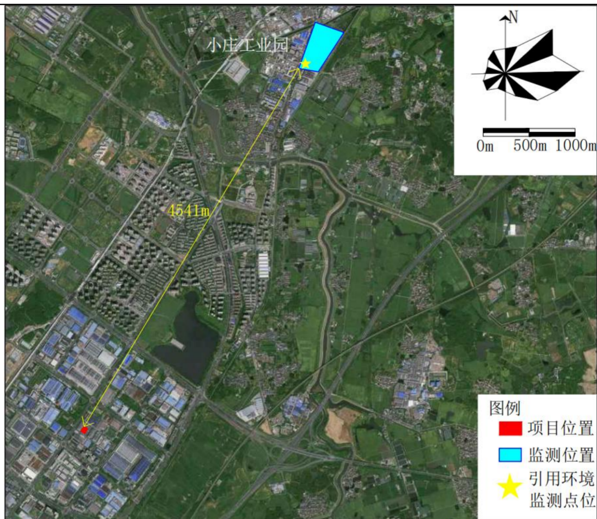
图 3-1 本项目与引用点位相对距离图
