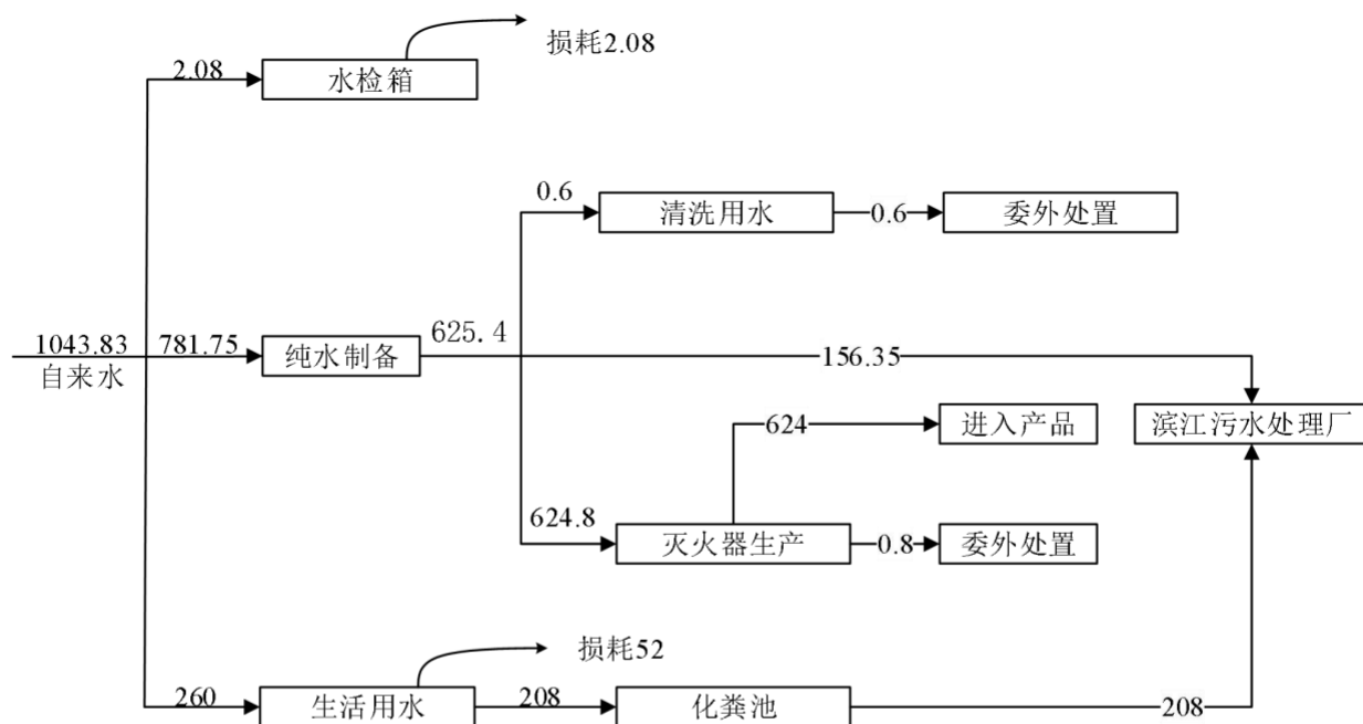
图 2-1 本项目给排水平衡图 单位: t/a
