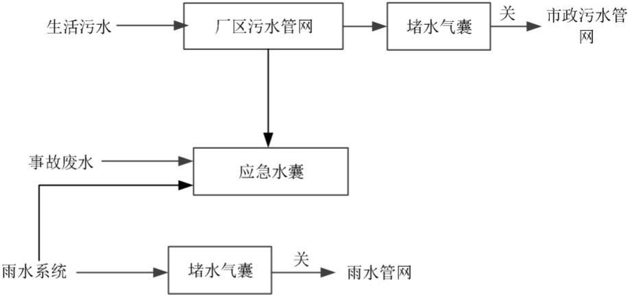
图4-1 废水防范、处理示意图
