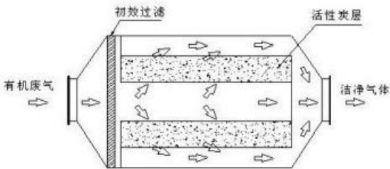
图 4-2 活性炭吸附装置结构图
