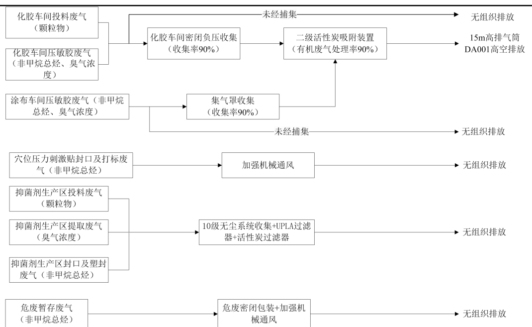
图 4-1 本项目废气收集治理走向流程图
