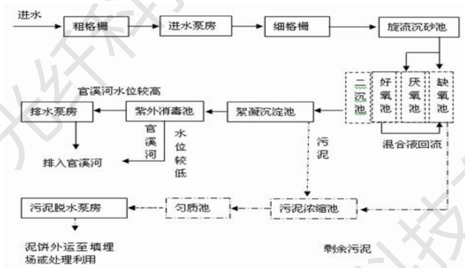
图 4-1 高淳新区污水处理厂工艺流程图
