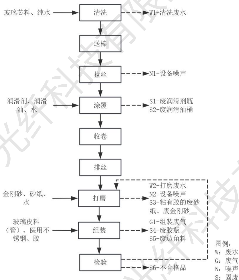
图 2-3 医用电子光纤内窥镜生产工艺流程图及产污环节
