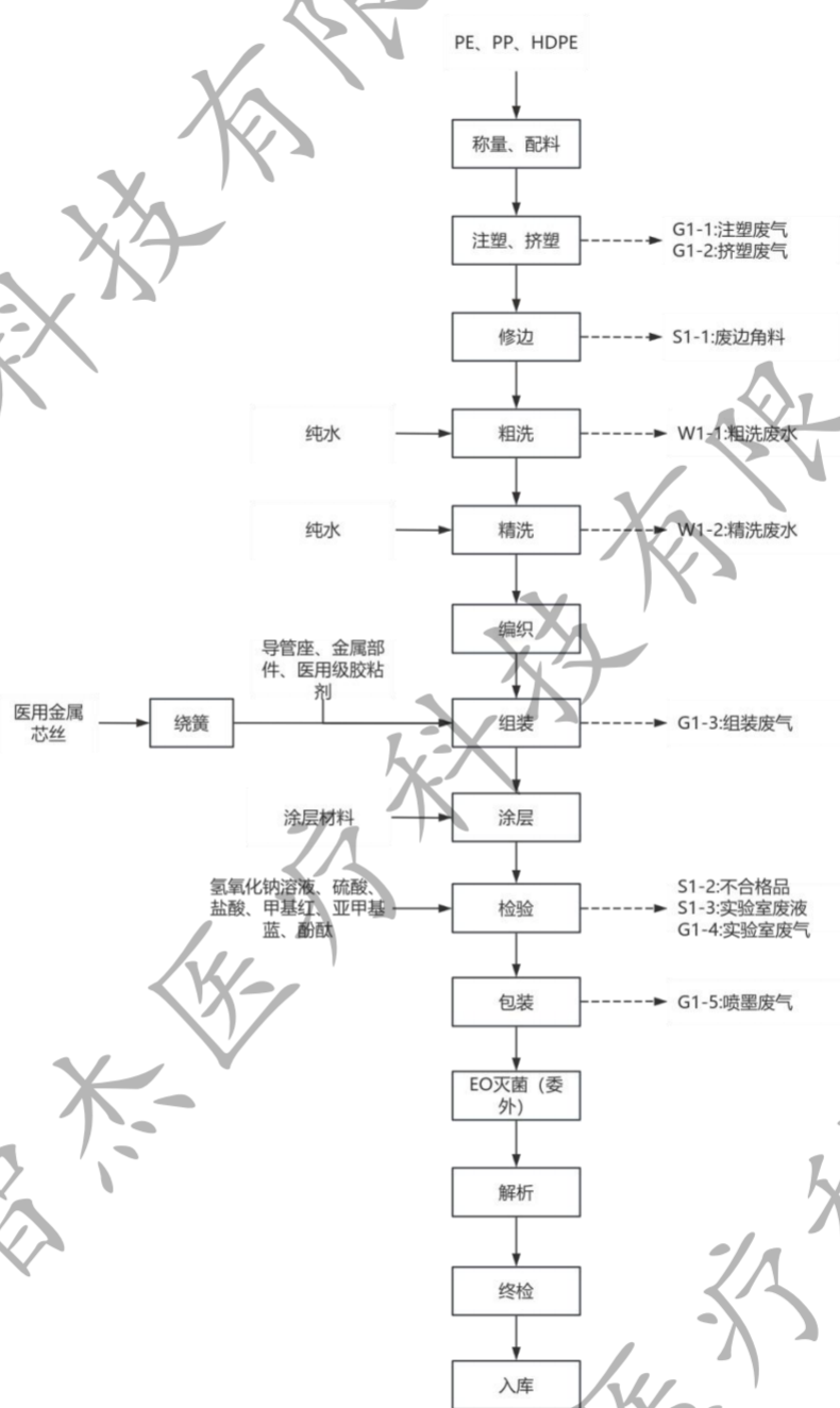
图 2-2 项目多功能球囊、穿刺针、医用导丝、神经阻滞针、吻合器、缝合器、负压引流瓶、冲洗导管、骨科外固定、中段尿液采集器生产工艺流程图
