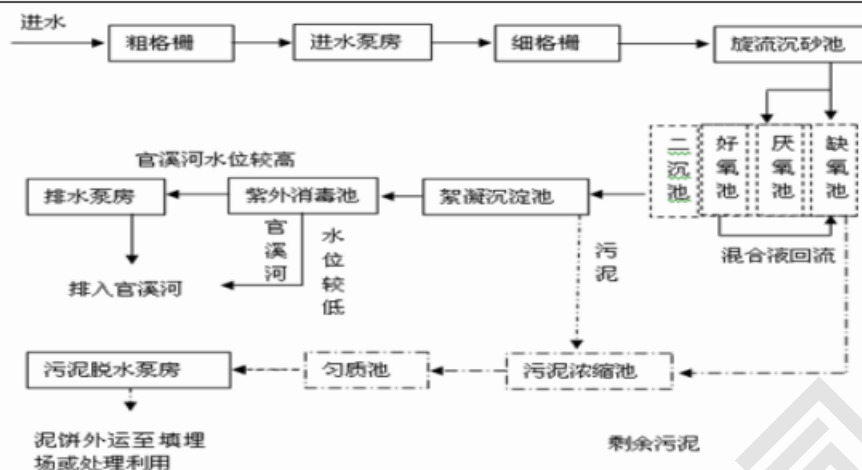
图 4-1 高淳新区污水处理厂工艺流程图
