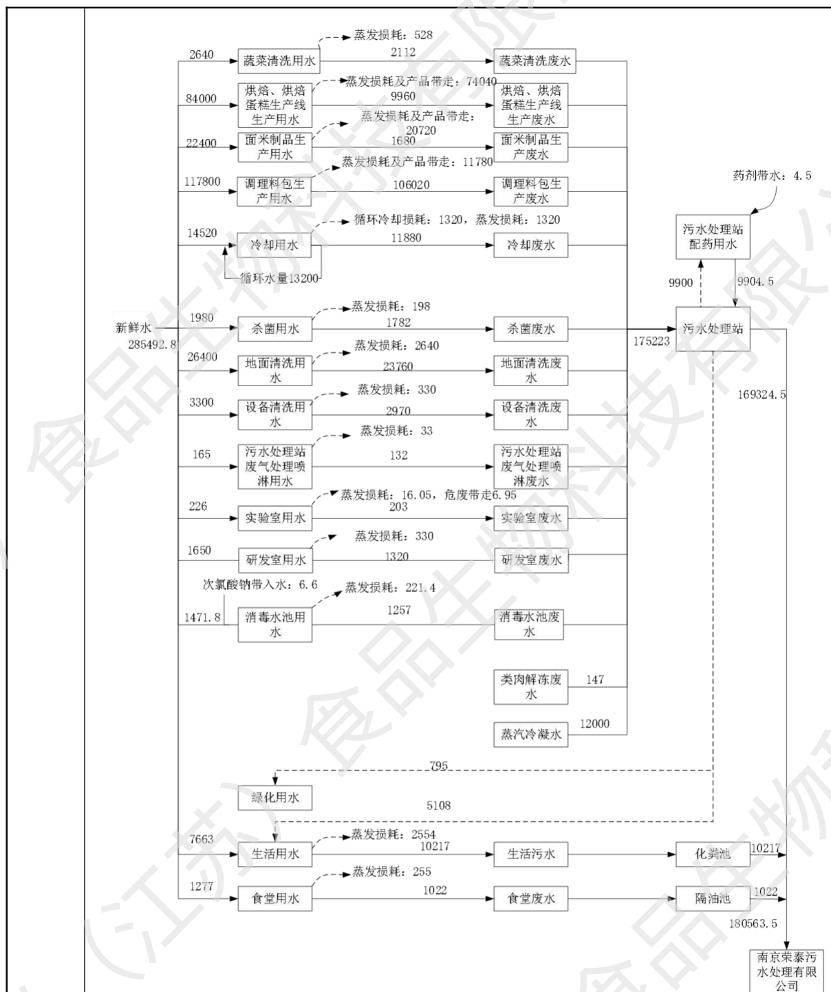
图 2-1 水平衡图 单位: t/a
