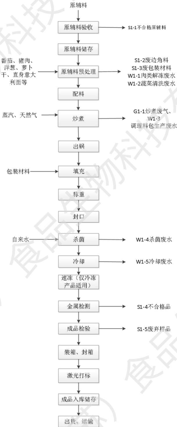
图 2-2 调料料包生产线工艺流程图
