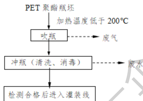
图 2-11 PET 制瓶工艺流程图及产污环节
