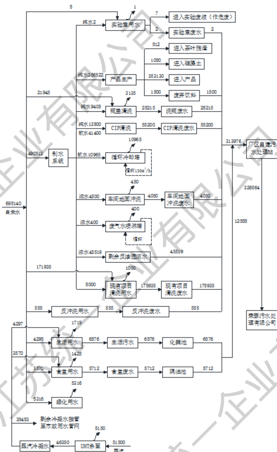
图 2-4 项目建成后全厂水平衡图
