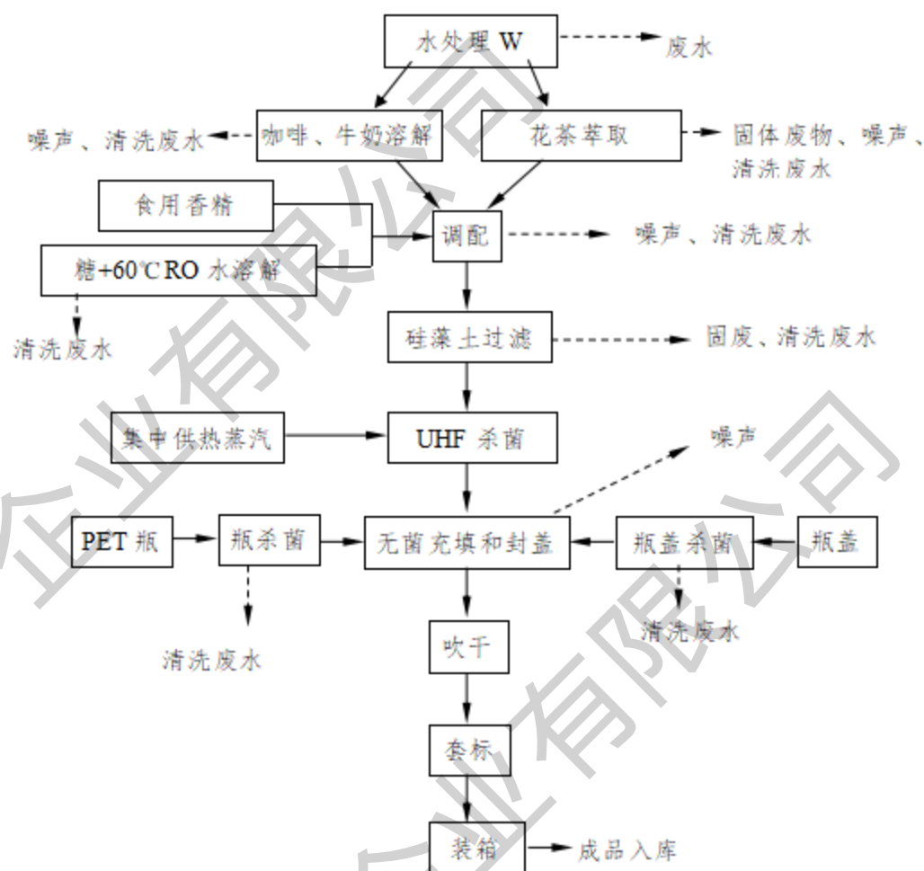
图 2-10 咖啡、奶茶等饮料生产工艺流程及产污环节
