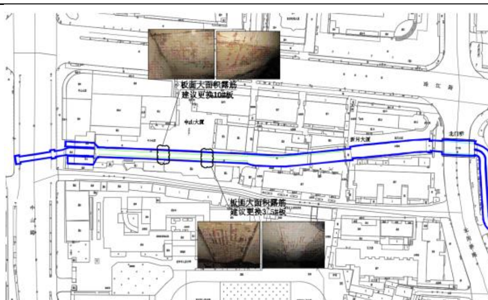
图 2.3-3 干河沿暗涵平面位置示意图
