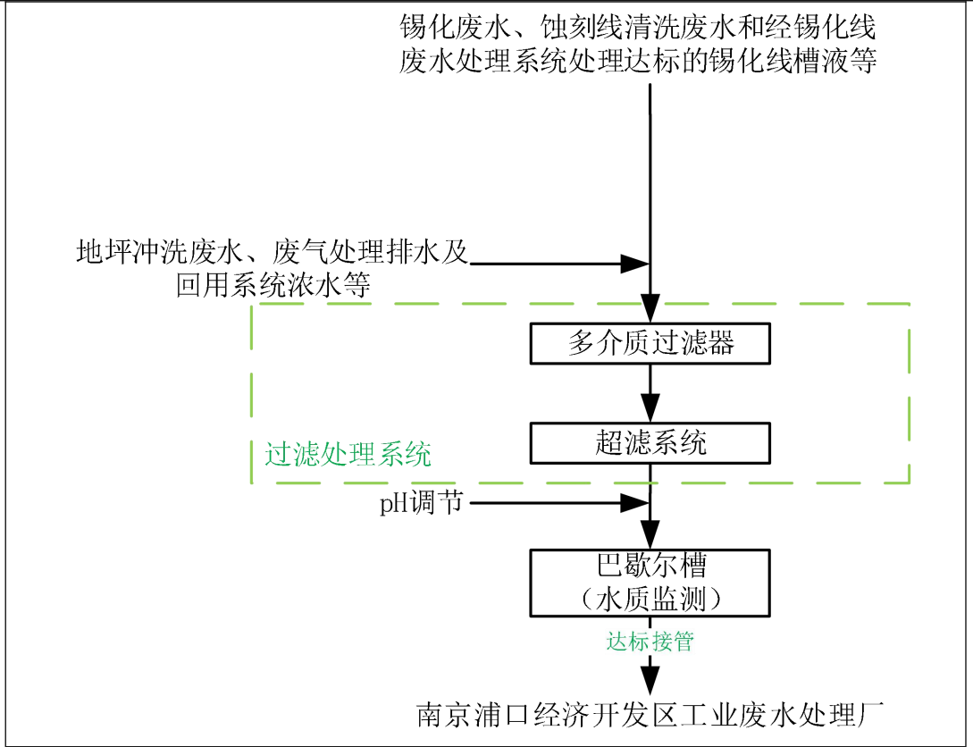
图 4-6 本次项目依托的厂区综合废水处理系统工艺流程示意图
