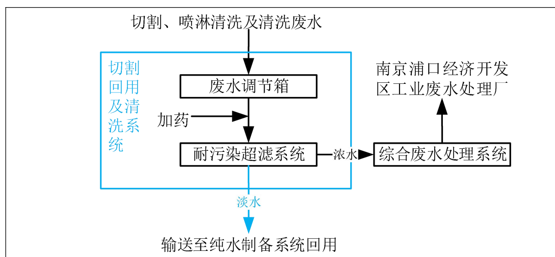
图 4-4 本次项目依托的切割及清洗回用系统工艺流程示意图
