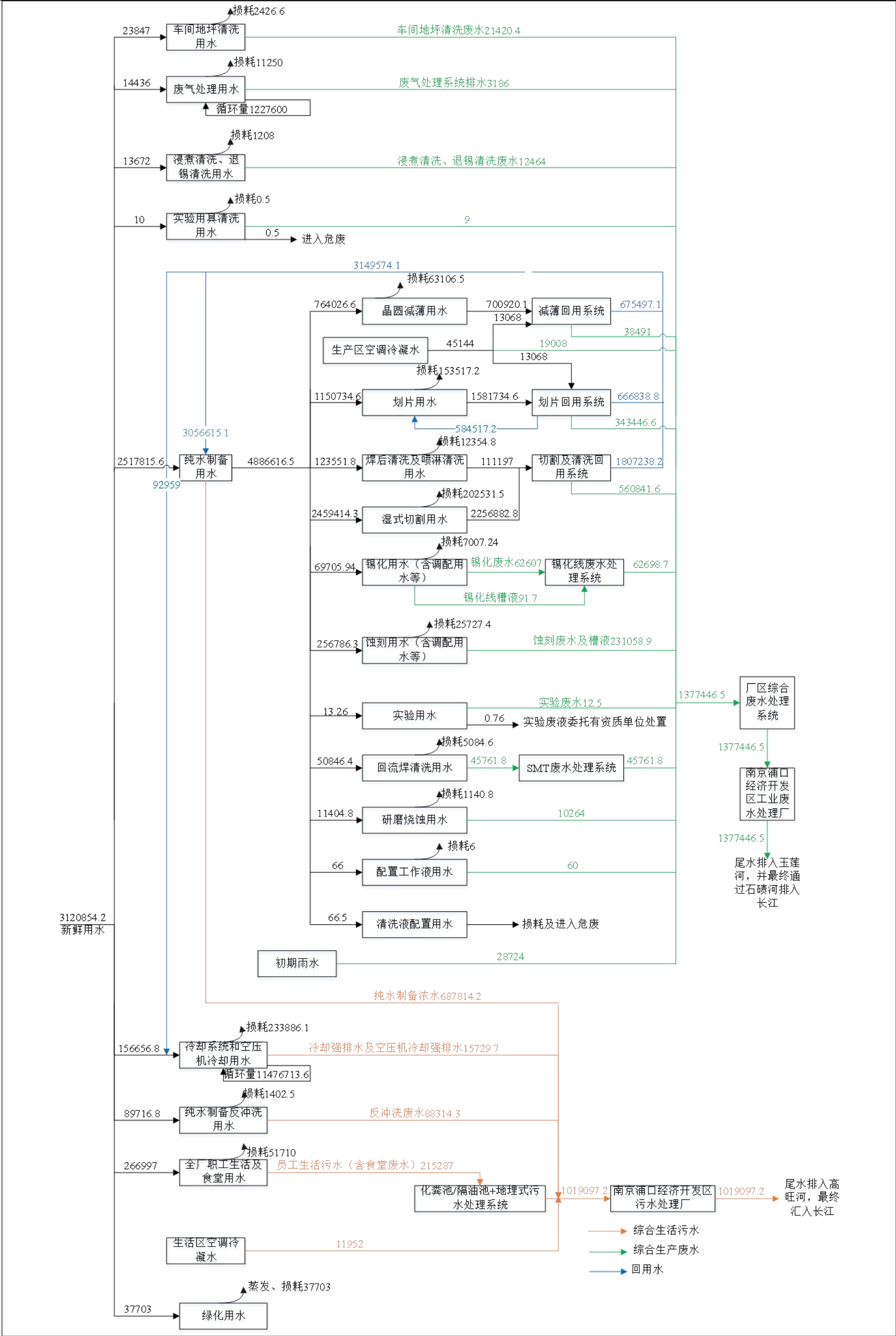
图 2-2 本次项目建成后全厂水平衡图 (单位 t/a)
