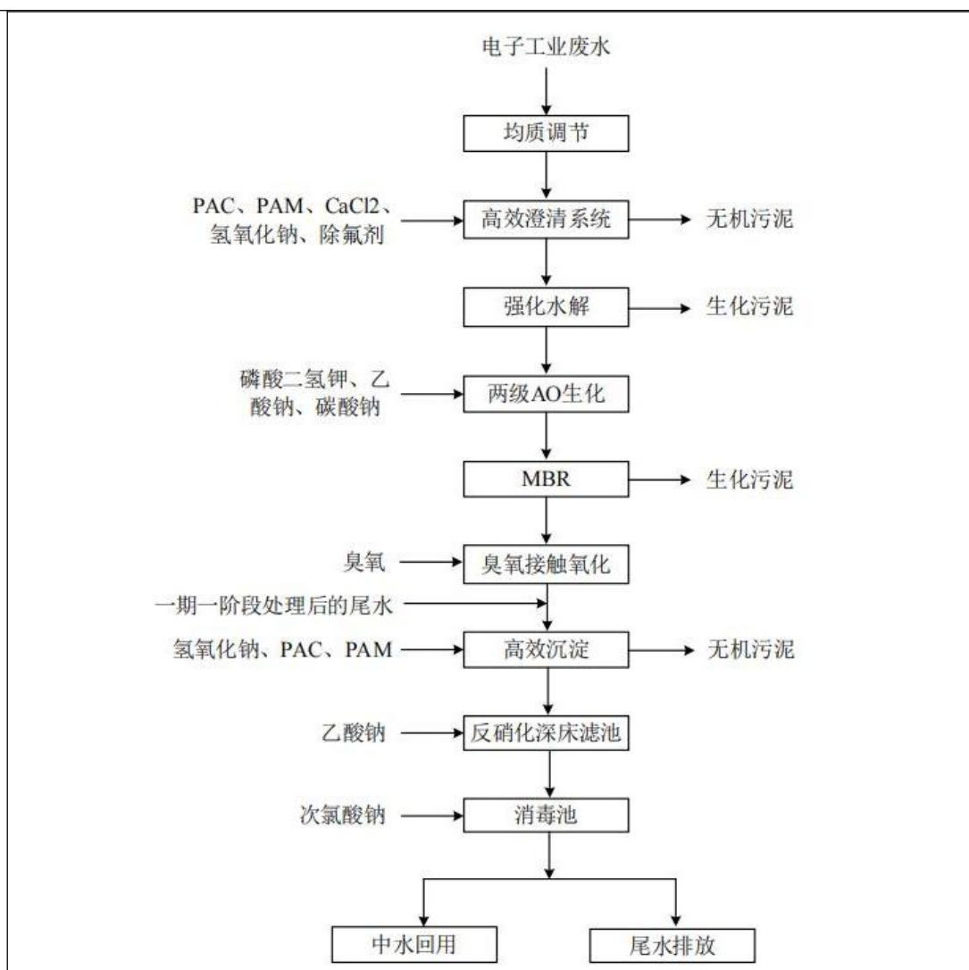
图 4-7 南京浦口经济开发区工业污水处理厂（一期一阶段）污水处理工艺流程图
