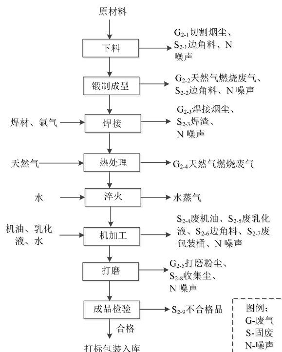
图 2-8 锻件类产品生产工艺流程图
