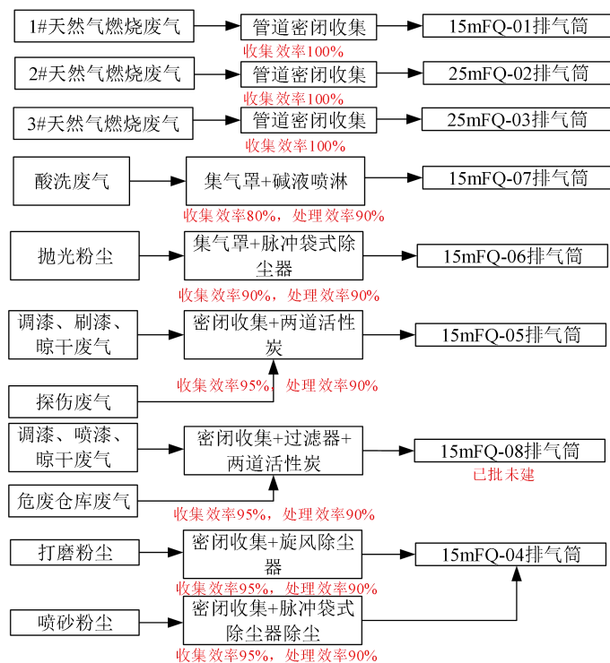
图 2-11 废气处理工艺流程图
