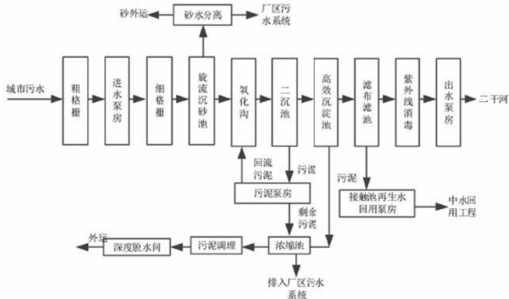
图 4-2 南京溧水东屏污水处理厂处理工艺流程图
