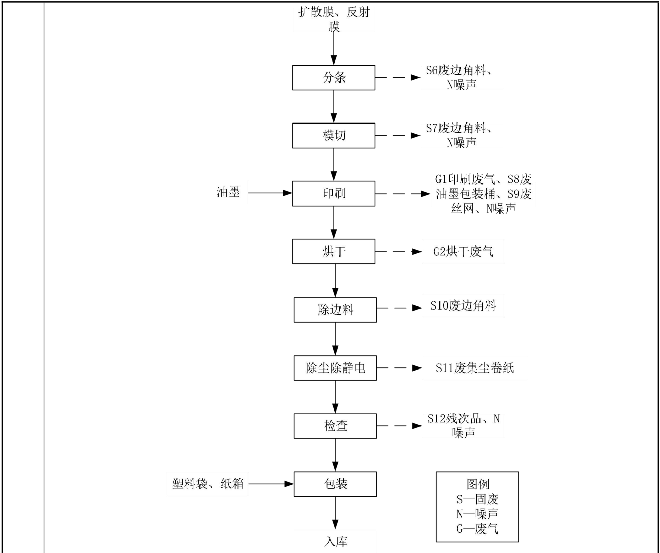
图 2-3 印刷膜片生产工艺流程图
