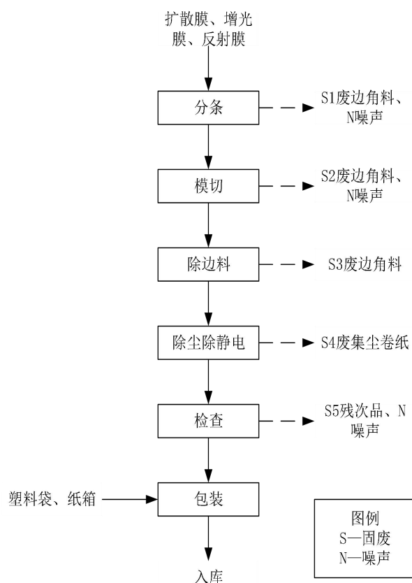
图 2-4 非印刷膜片生产工艺流程图
