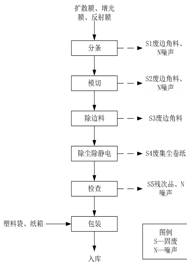
图 2-2 非印刷膜片生产工艺流程图
