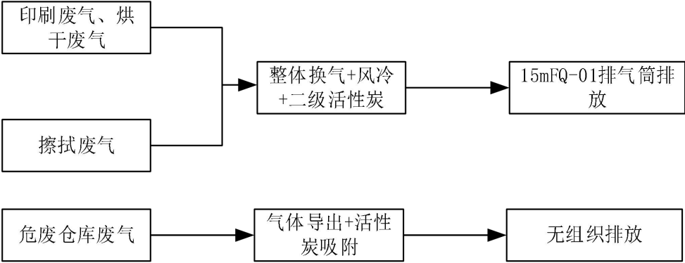
图 4-1 运营期废气治理措施图
