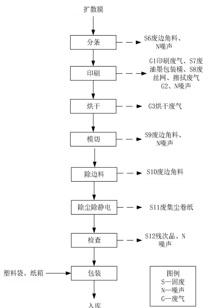
图 2-5 印刷膜片生产工艺流程图
