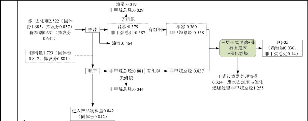
图 2-2 建设项目喷漆物料平衡图 单位: t/a 灌漆和补漆平衡:
