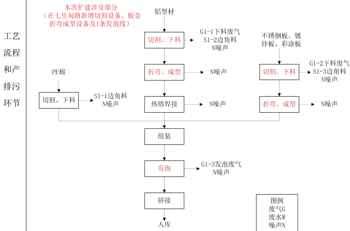
图 2-5 中央空调检修门工艺流程及产污环节图
