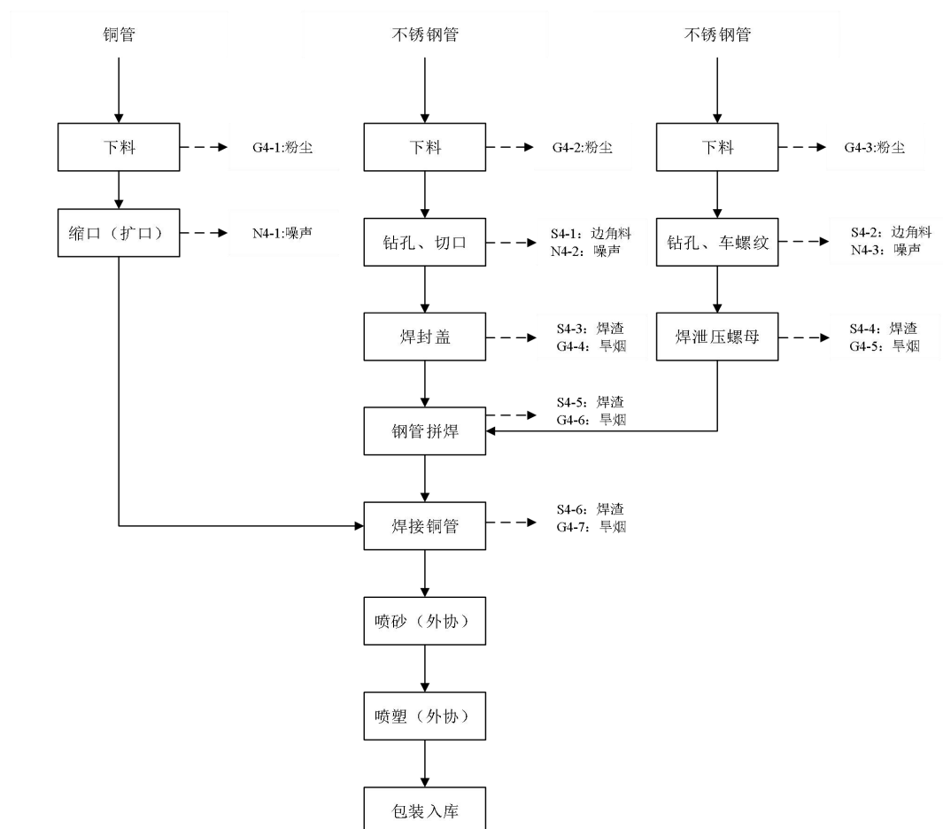
图 2-10 空调集水管生产线工艺流程图
