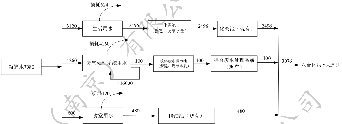
图 2-3 一期工程实施后水平衡图（单位：m³/a）
