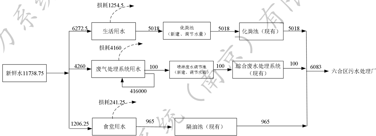
图 2-4 二期工程实施后水平衡图（单位：m³/a）
