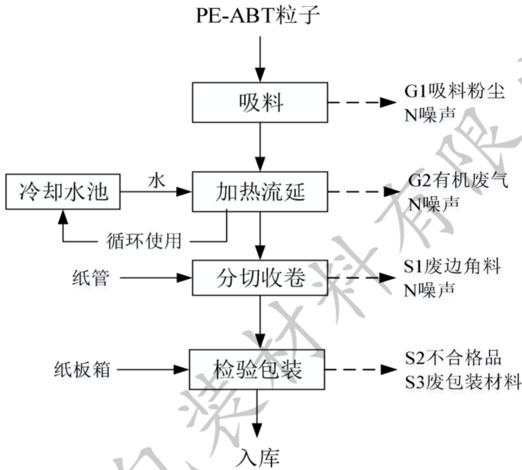
图 2-3 包装膜生产工艺流程及产污节点图
