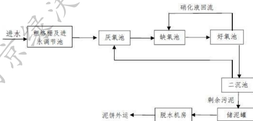
图 4-1 横梁大仇污水处理厂处理工艺流程图
