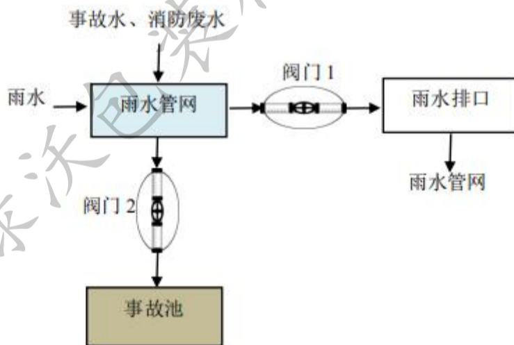
图 4-3 事故水、消防废水收集排放管控示意图
