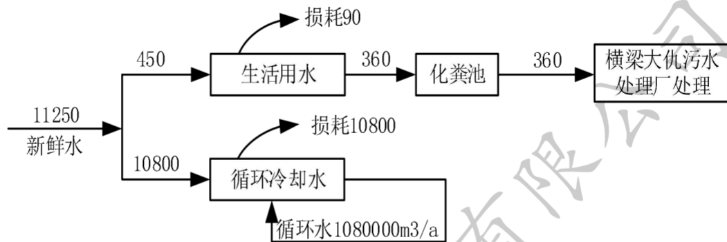
图 2-1 本项目给排水平衡图 (t/a)
