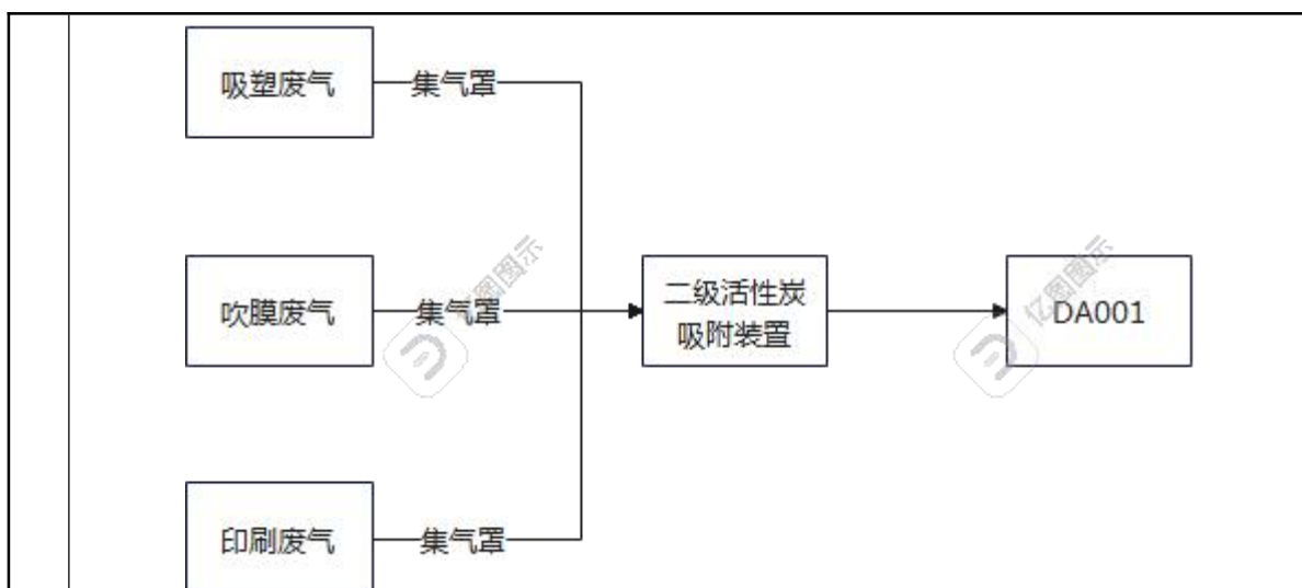
图 4-1 项目废气治理流程图
