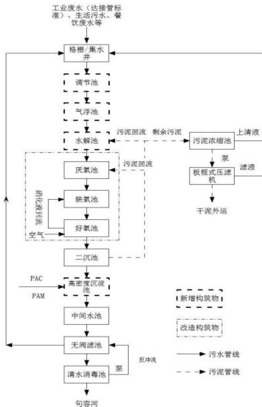
图 4-4 湖熟集镇污水处理厂处理工艺流程图
