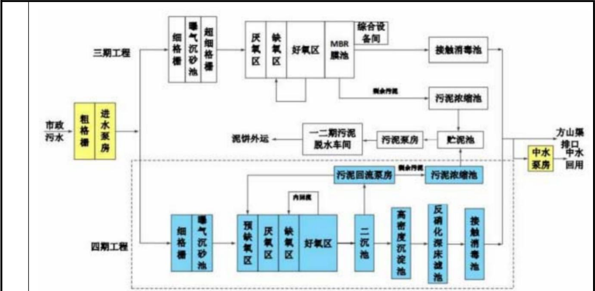
图 4-2 江宁科学园污水处理厂三期工艺流程图
