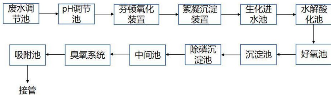
图 4-1 小镇南区污水处理站废水处理工艺流程图
