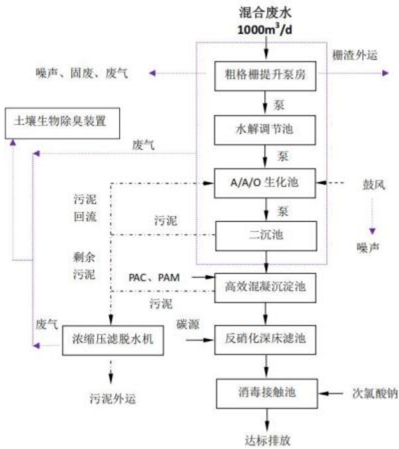
图 4-1 索墅污水处理厂工艺流程图
