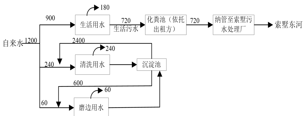
图 2-2 项目全厂水平衡图（单位：t/a）
