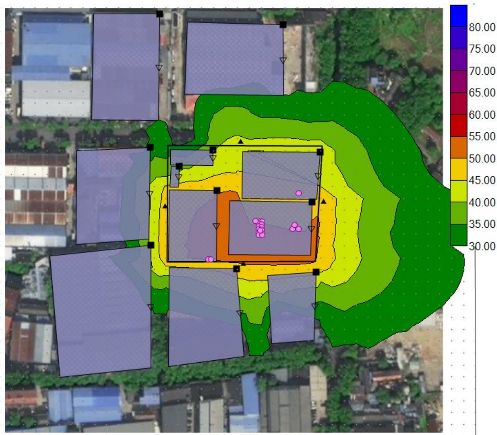
图 4-3 噪声影响贡献值等声级线图
