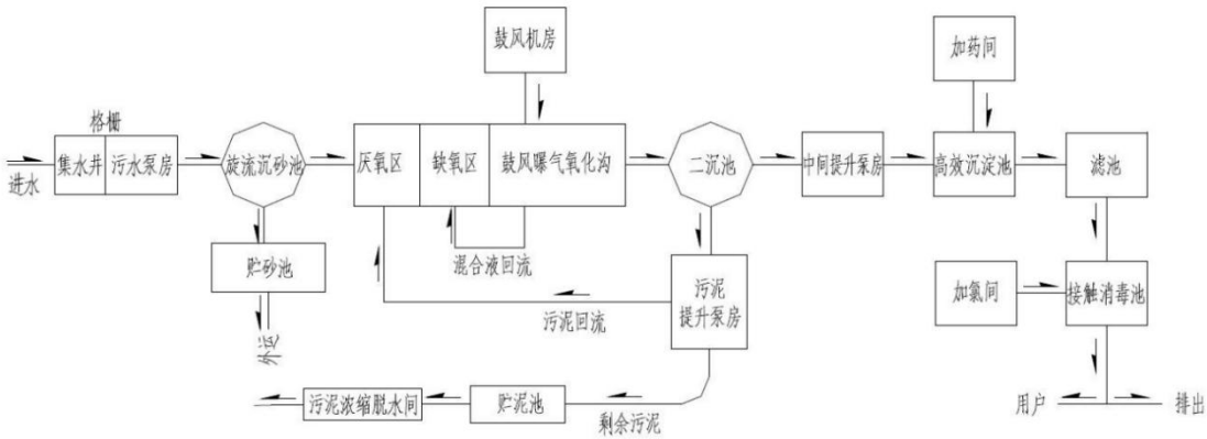
图 4-2 污水处理厂处理工艺流程图
