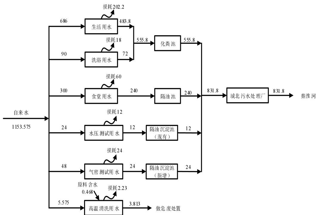
图 2-2 本项目建成后全厂水平衡图 (t/a)
