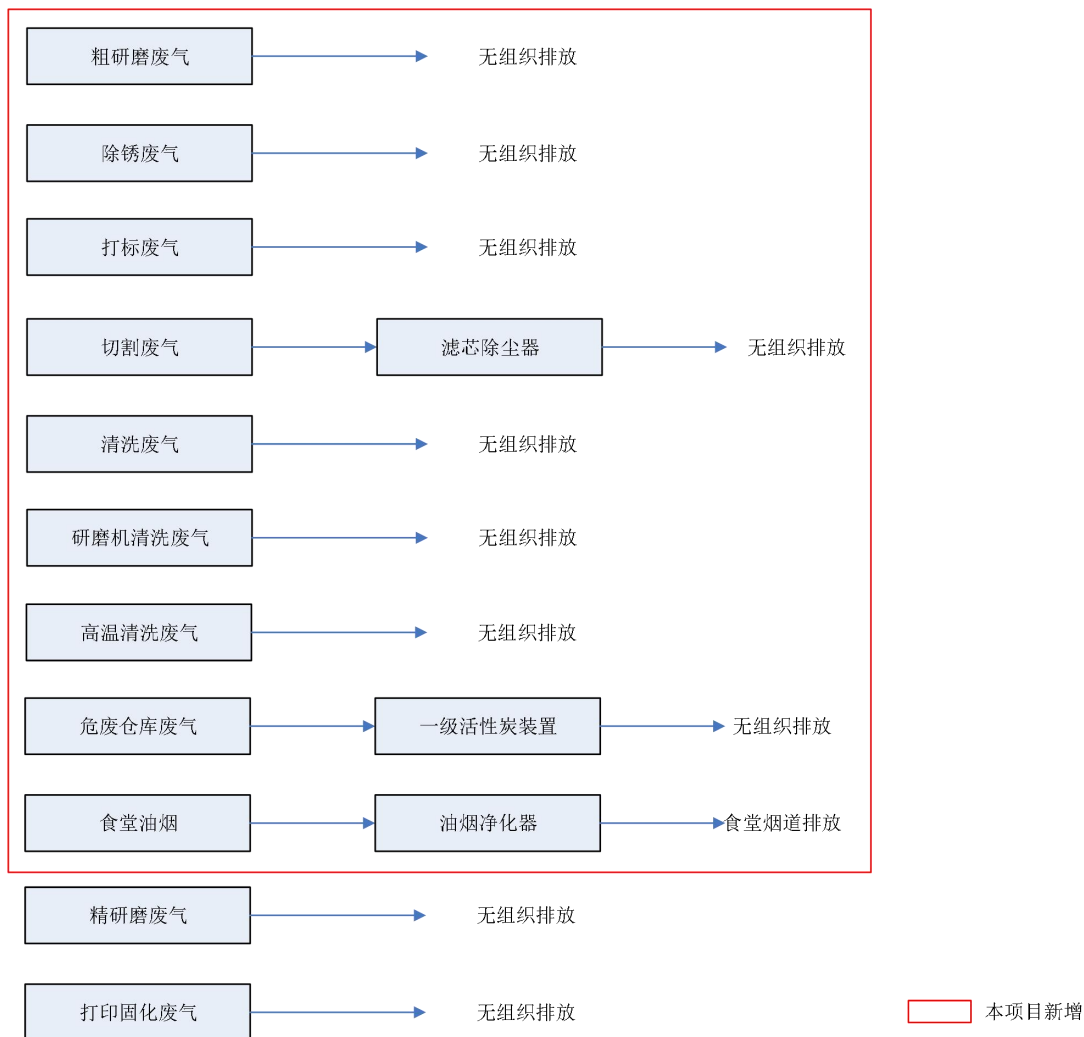
图 4-1 全厂废气收集处理示意图
